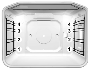
съемные направляющие
